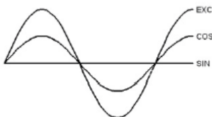
图 5.5: 电机旋转位置为 0
